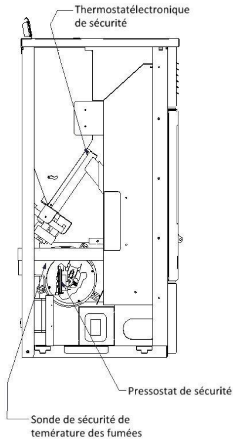
Figure 3 Emplacement des capteurs de commande et des dispositifs de sécurité
